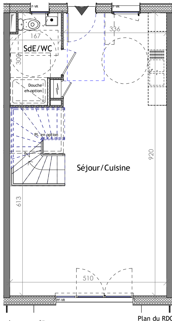
Plan du RDC
